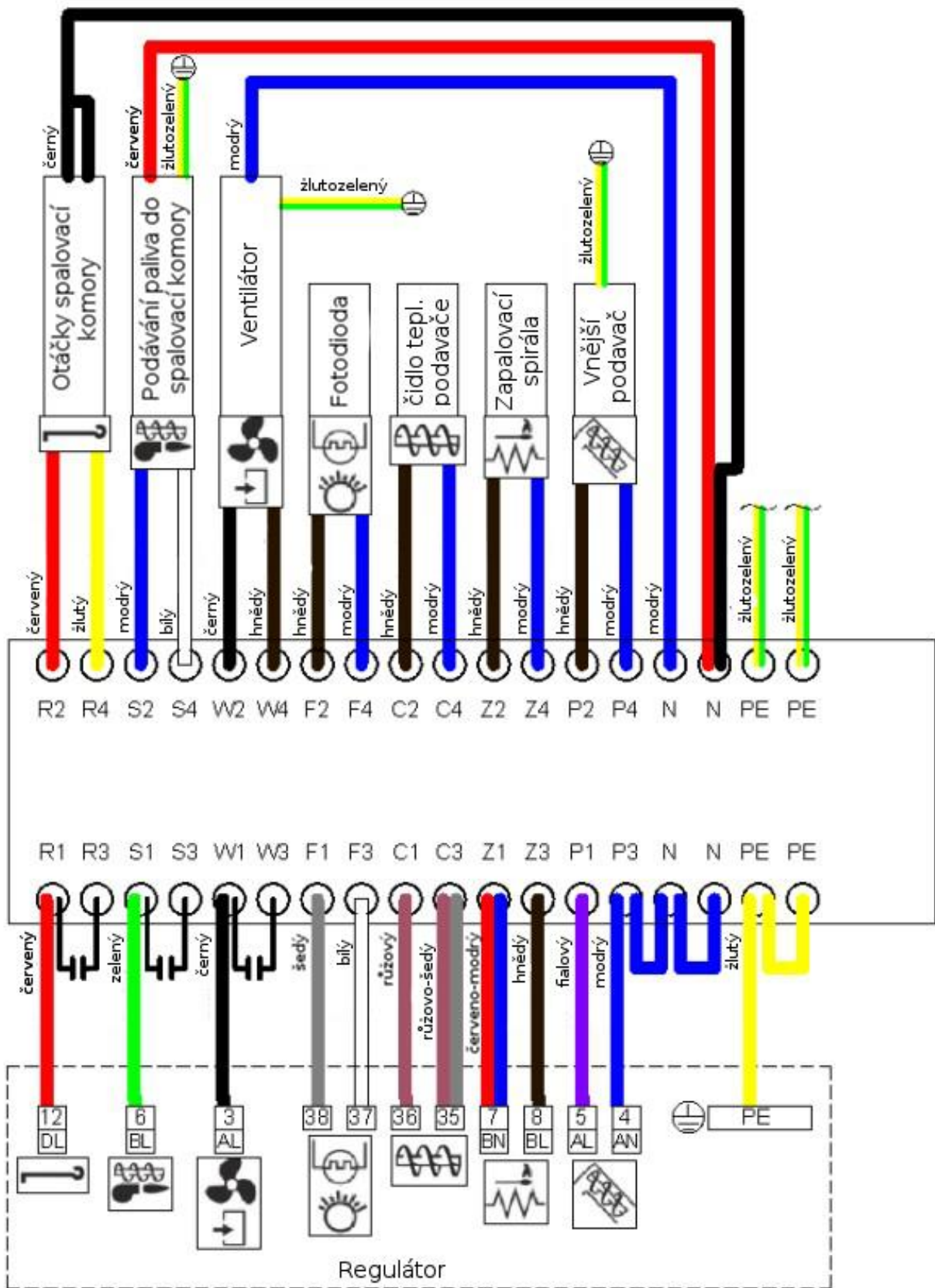
Obr. č. 17 Elektrické schéma zapojení hořáku
